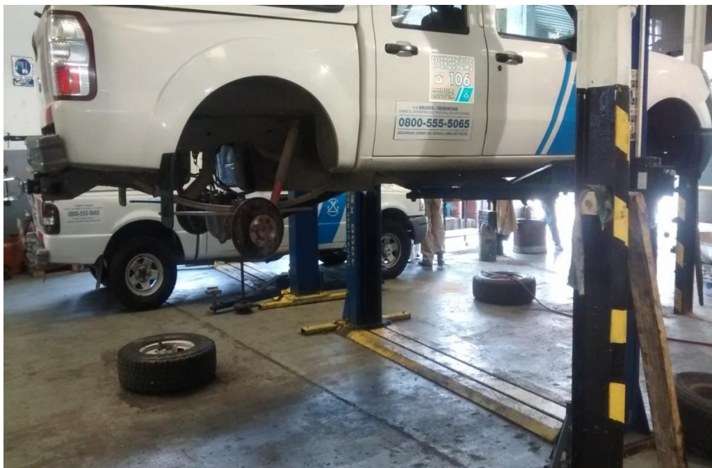
FIG 4: FORD RANGER 3.0. REPARACIÓN COMPLETA DE FRENOS Y CAMBIO DE RODAMIENTOS DE PALIER – SECCIÓN MECÁNICA TA.GE.RE.AU.
