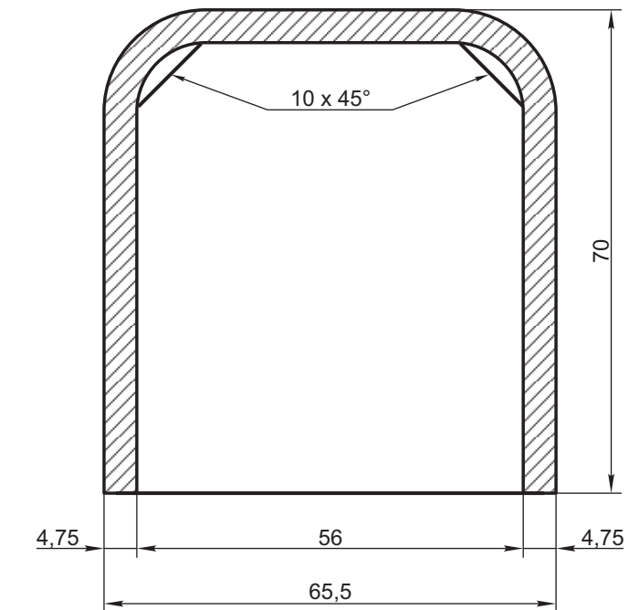
CORTE CC
