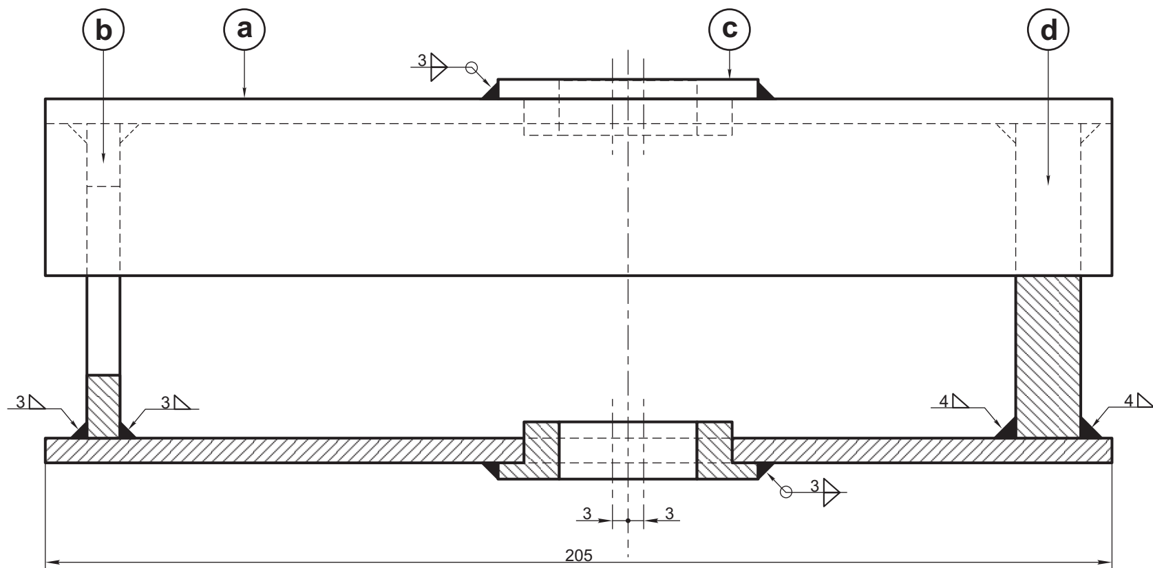
CORTE AA
