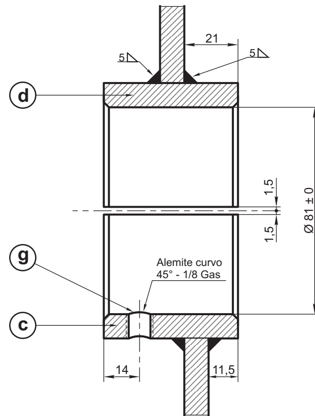
CORTE BB (S/Escala)
