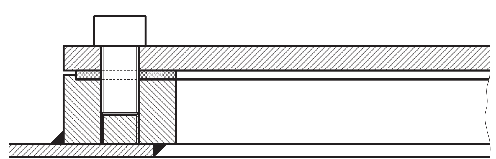
CORTE A-A Esc. 1:1
