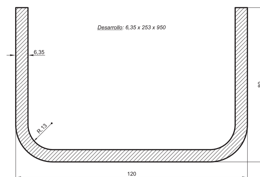
CORTE A-A Esc. 1:1
