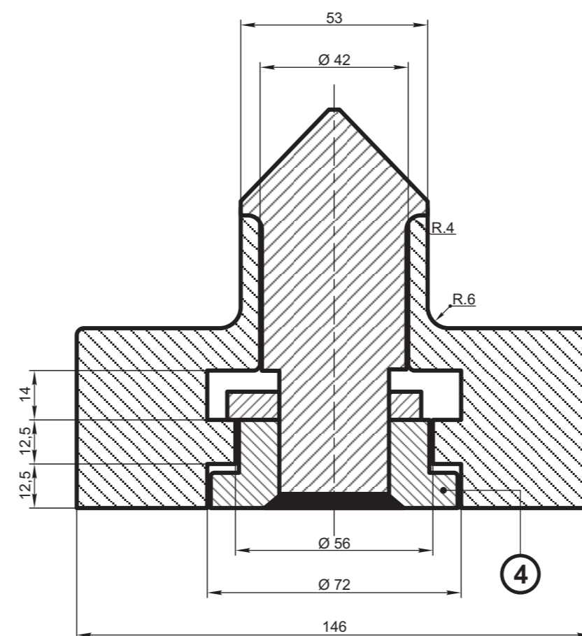
CORTE A-A
