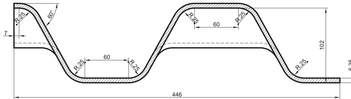
Antes de plegar pestaña (Esc. 1:2,5)
