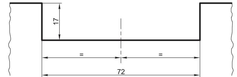
Detalle del recorte para librar bisagras (Esc. 1:1)
