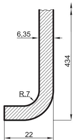
Detalle de la pestaña (Esc. 1:1)
