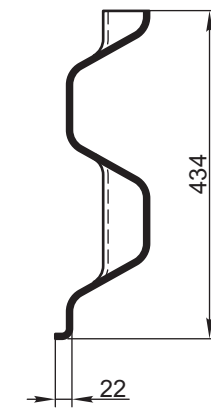
CORTE A-A
