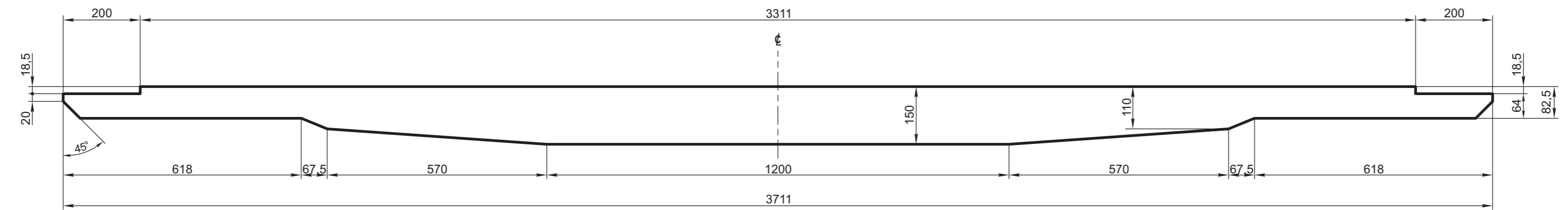
Desarrollo longitudinal
