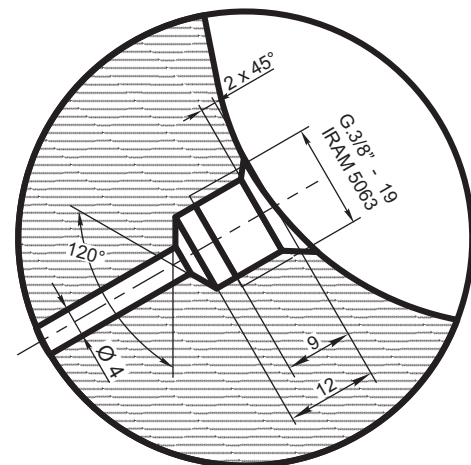
DETALLE "1" (Esc. 1:1)
