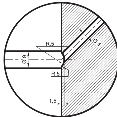
DETALLE "2" (Esc. 1:1)
