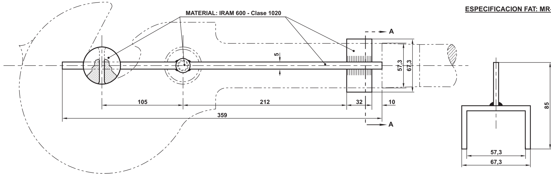
CORTE A-A
