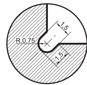
DETALLE 1 (Esc. 5:1)
