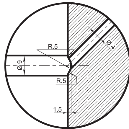
DETALLE "2" (Esc. 1:1)
