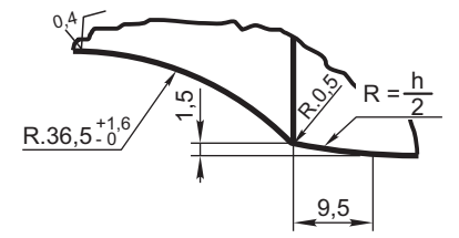
DETALLE "X" (Esc. 1:1)
