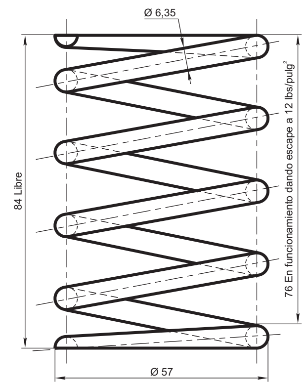
PIEZA N° 849/B (Esc. 1:1)
