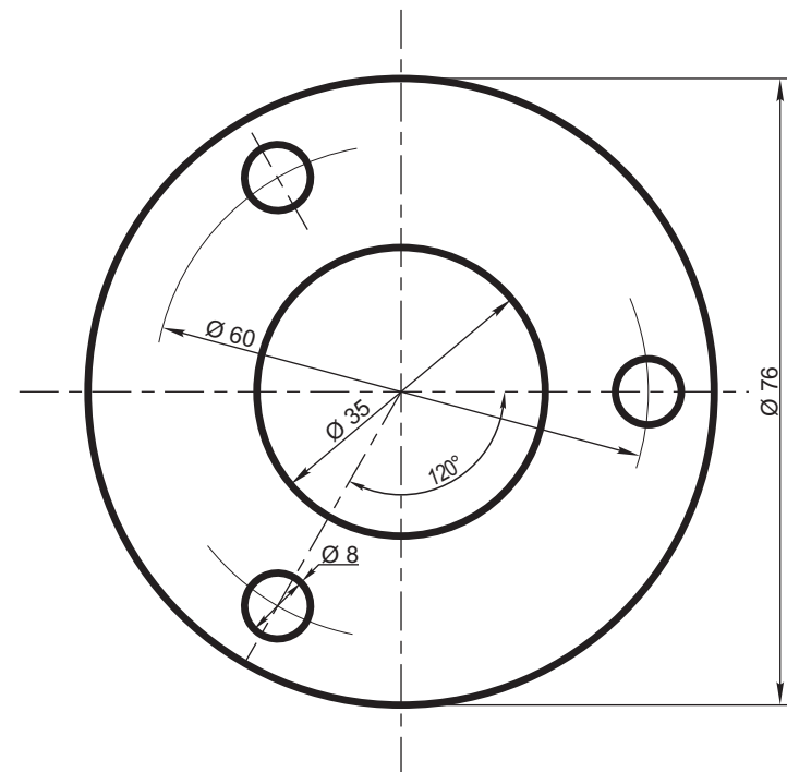
PIEZA N° 757
