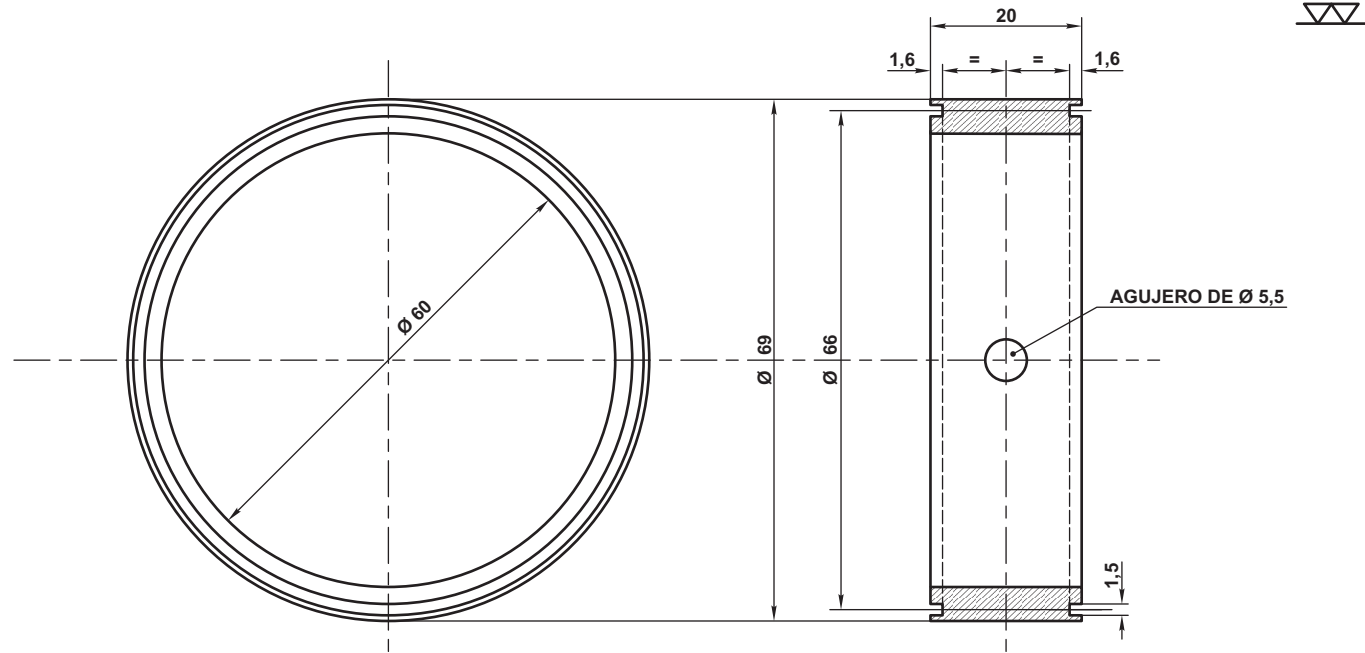
PIECE N° 732 PIEZA
