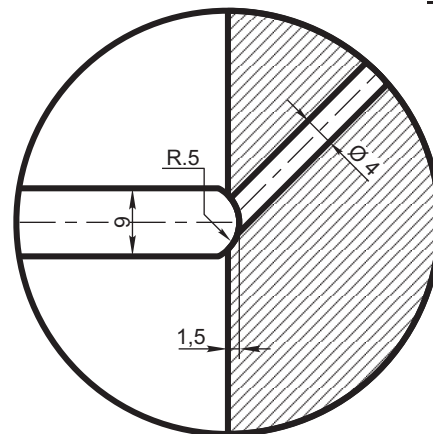
DETALLE "2" (Esc. 1:1)
