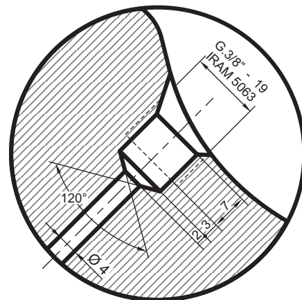
DETALLE "1" (Esc. 1:1)
