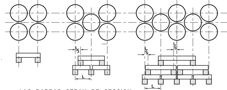
LAS BARRAS SERAN DE SECCION CUADRADA DE 25 x 25 mm Y SU LONGITUD SE ADECUARA AL DISEÑO DEL BOGIE.
