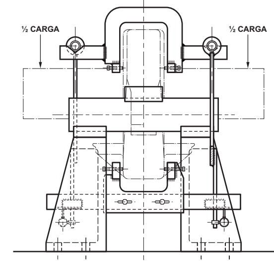
DISPOSITIVO SUMULADOR DEL REPARTO DE CARGAS EN EL ASIENTO DE RESORTES
