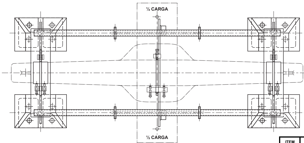
LAS BARRAS SERAN DE SECCION CUADRADA DE 25 x 25 mm Y SU LONGITUD SE ADECUARA AL DISEÑO DEL BOGIE.
