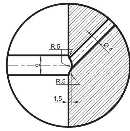
DETALLE "2" (Esc. 1:1)
