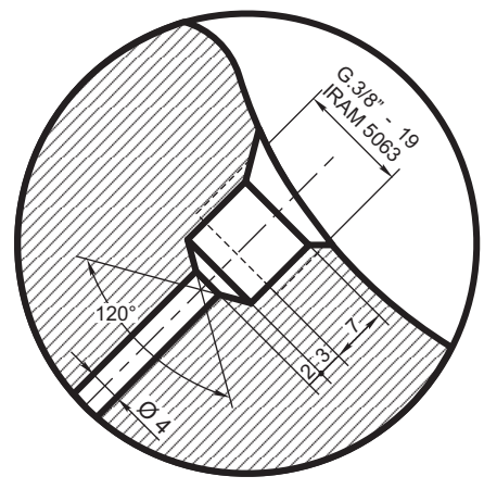
DETALLE "1" (Esc. 1:1)
