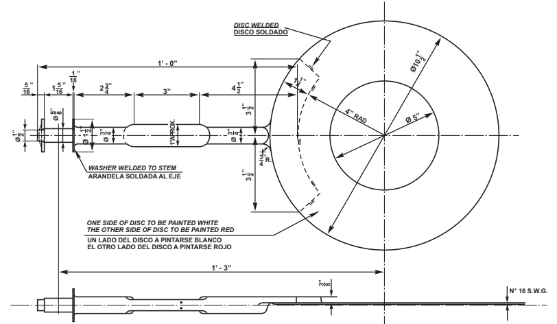
DETAIL OF DISC WITH STEM DETALLE DEL DISCO CON EJE PIECE N° 426/A PIEZA N° 426/A
