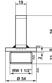
DETALLE B
