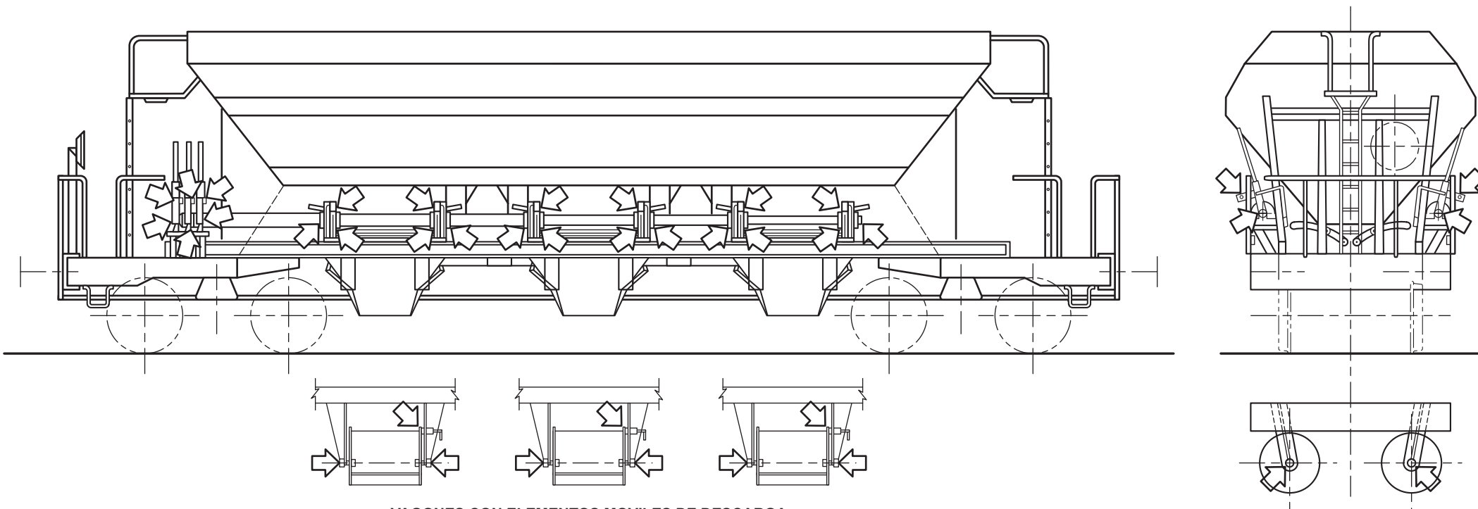
VAGONES CON ELEMENTOS MOVILES DE DESCARGA
