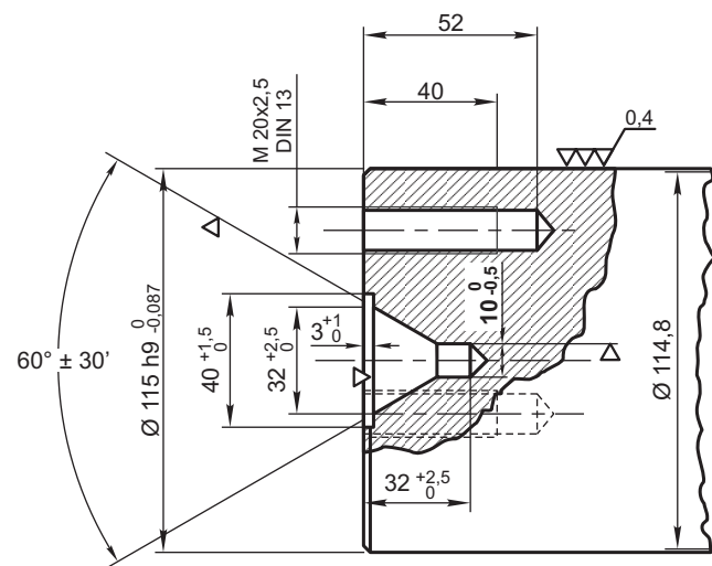
DETALLE E
