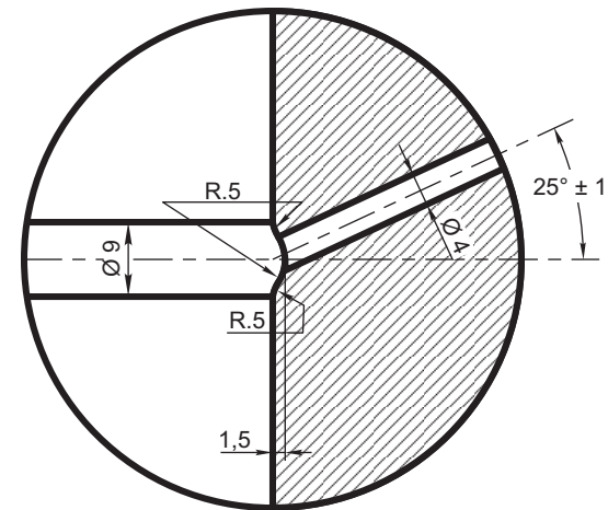
DETALLE "2" (Esc. 1:1)
