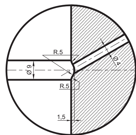
DETALLE "2" (Esc. 1:1)
