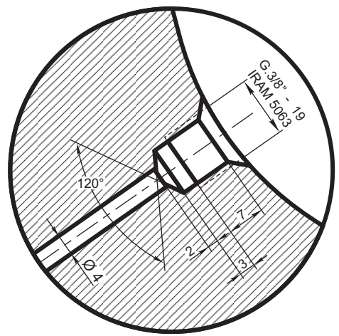
DETALLE "1" (Esc. 1:1)
