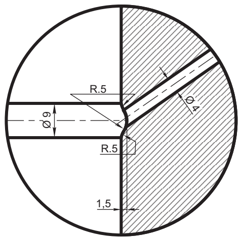
DETALLE "2" (Esc. 1:1)
