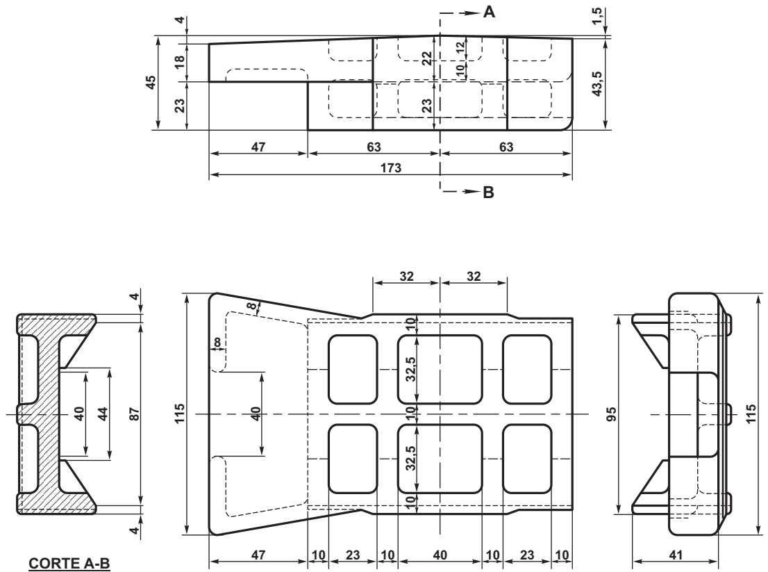
CORTE A-B
