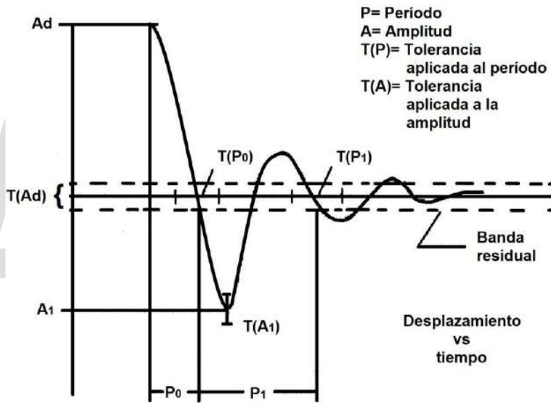
Figura 4.2B Respuesta con amortiguación crítica
