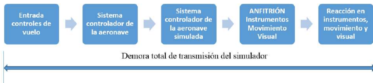
Figura 3.2G Tiempos de transmisión para simulación de aeronaves controladas por computador usando emulación de software de cajas negras de helicóptero
