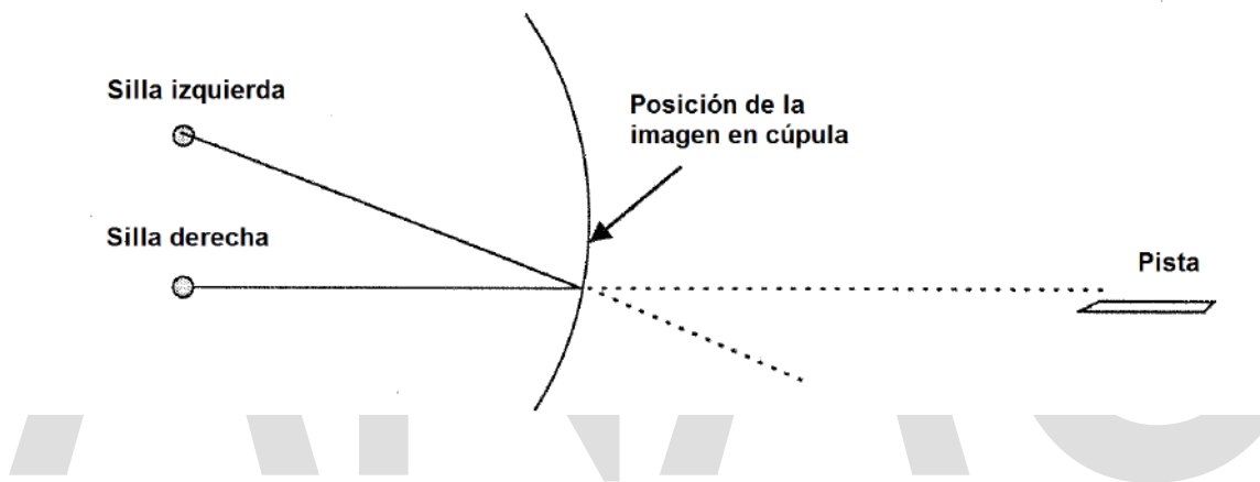
Figura 3.2K Visualización de la pista en una pantalla en cúpula
