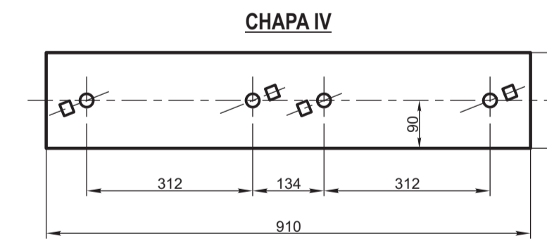
DIMENSIONADO DE CHAPAS DE ASIENTO Esc. 1:10
