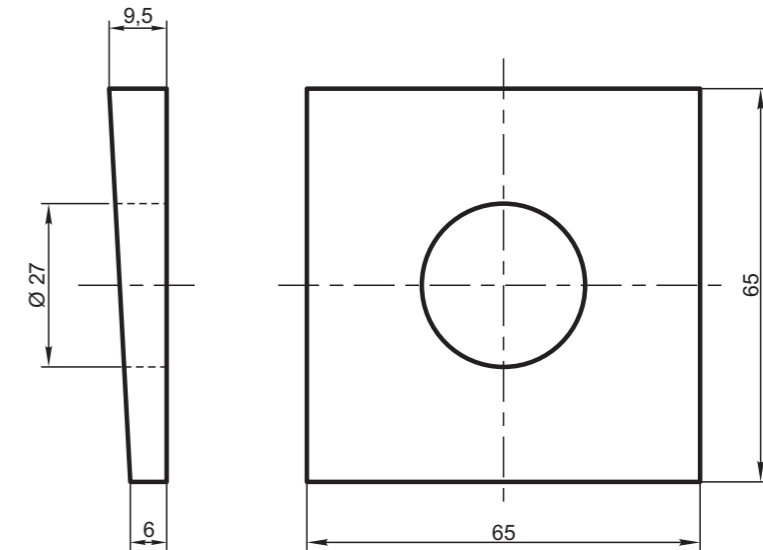
ARANDELA CUÑA
