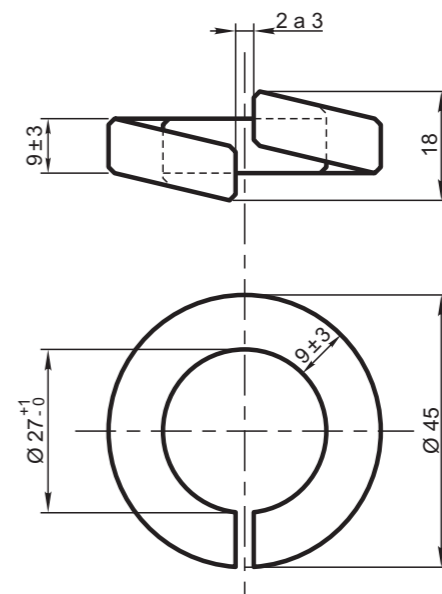
ARANDELA ELASTICA PARA BULON Ø 25,4
