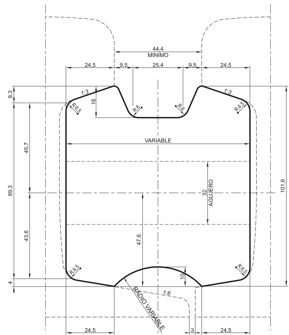
PERFIL TIPO DE PIEZAS DE DISTANCIA Esc. 1:1
