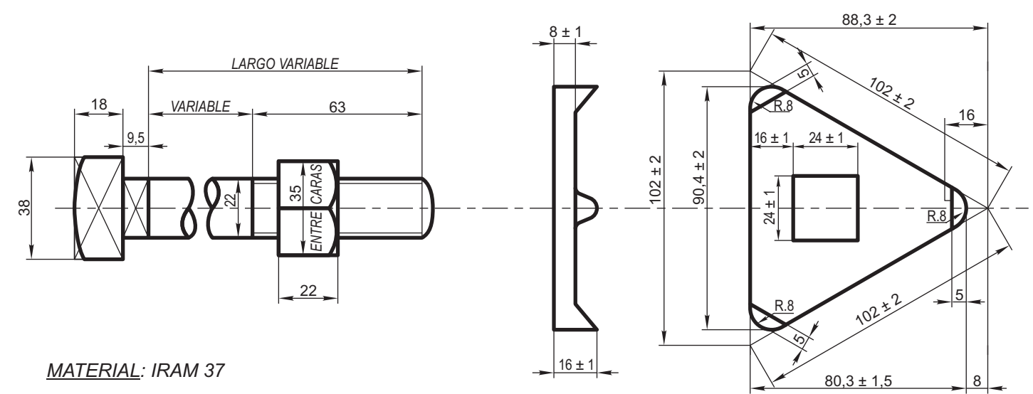
BULON PARA VIA TIPO "FANG" DESMONTABLE Esc. 1:2
