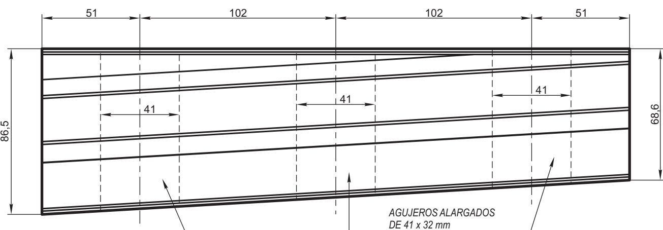
PIEZA DE DISTANCIA T.N. 9 T.N. 10 SIMETRICA Y OPUESTA Esc. 1:2
