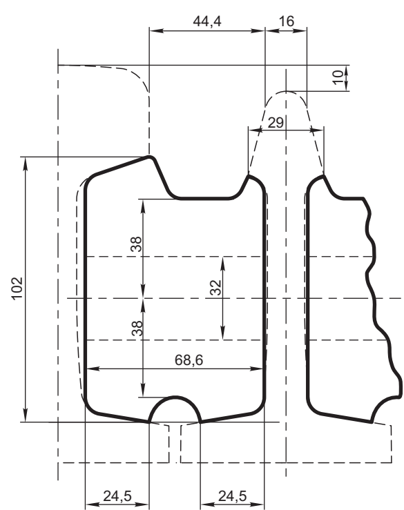
PERFIL TIPO DE PIEZAS DE DISTANCIA Esc. 1:1
