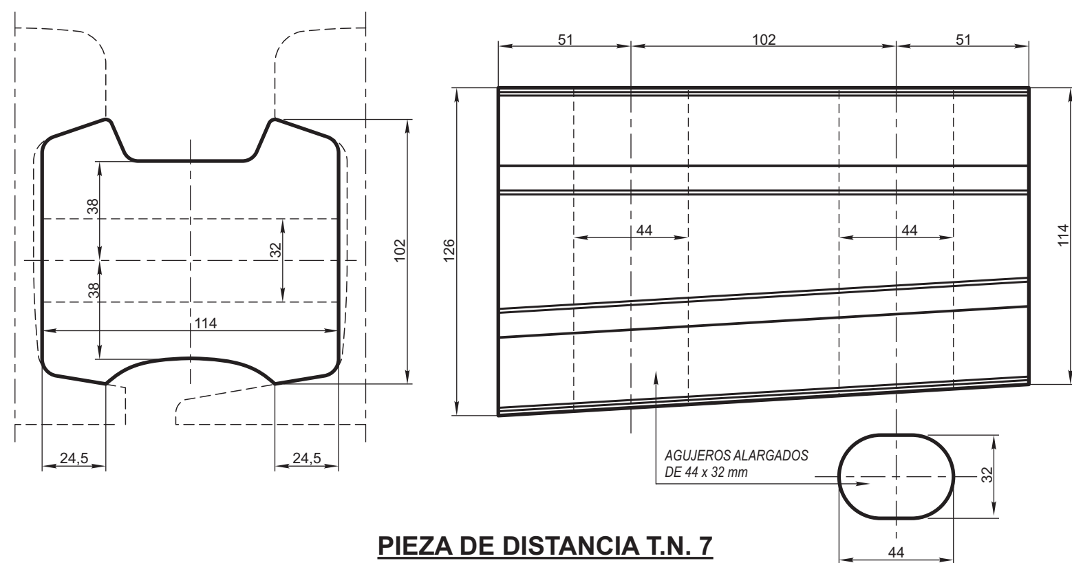
PIEZA DE DISTANCIA T.N. 7 T.N. 6 SIMETRICA Y OPUESTA Esc. 1:2
