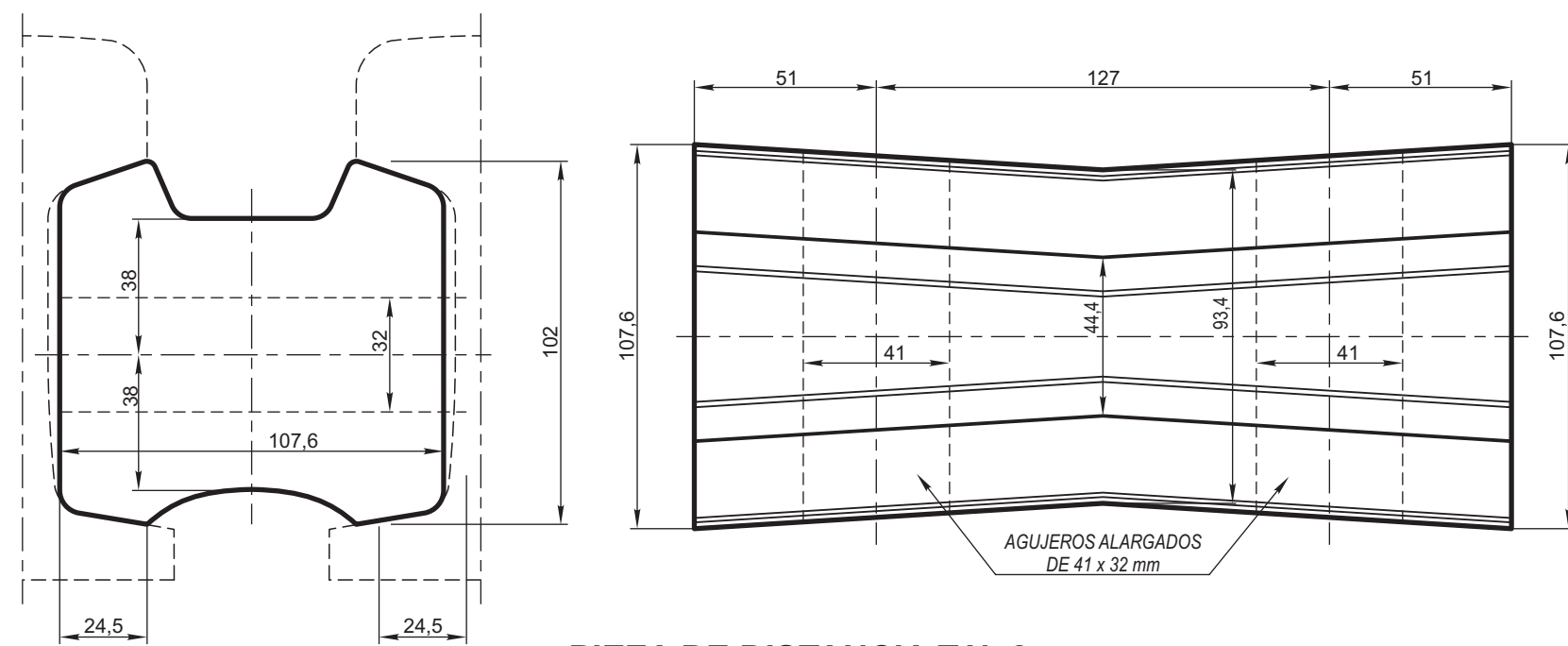
PIEZA DE DISTANCIA T.N. 8 Esc. 1:2
