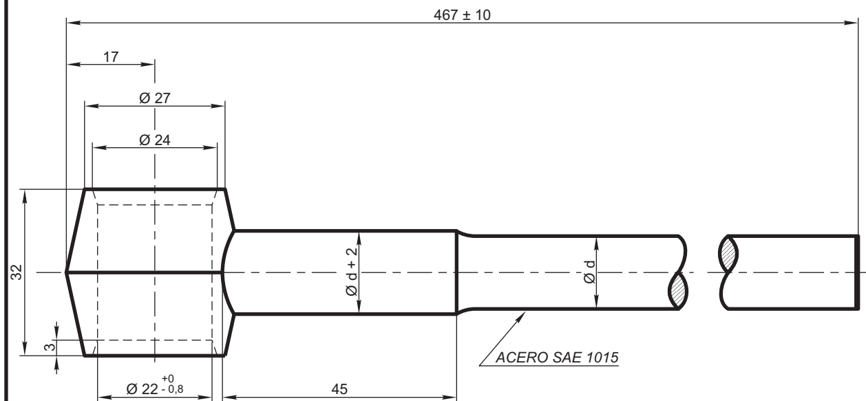
SECCION a - a
