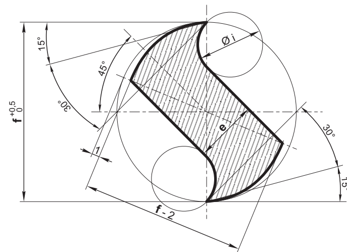
CORTE b-b Esc. 2:1
