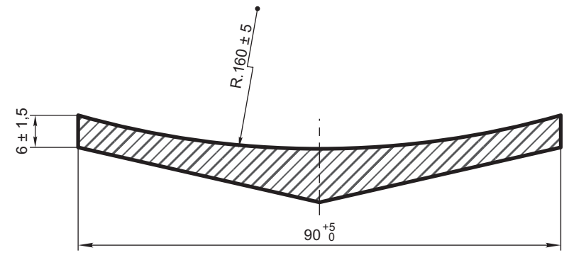
CORTE C-C
