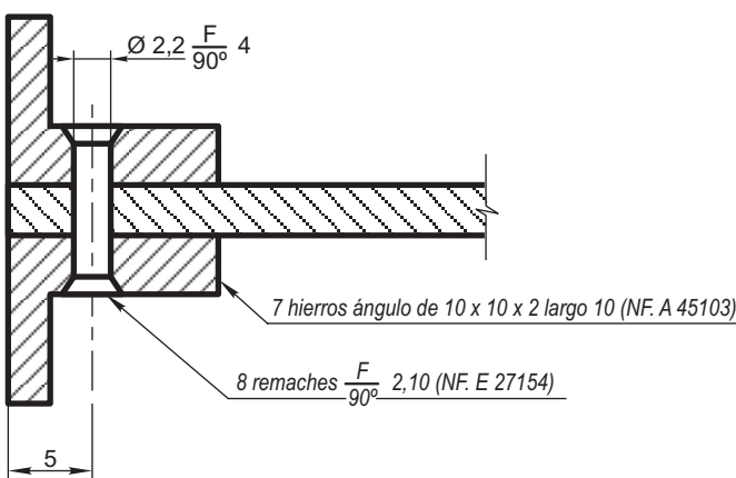
SECCION A-A
