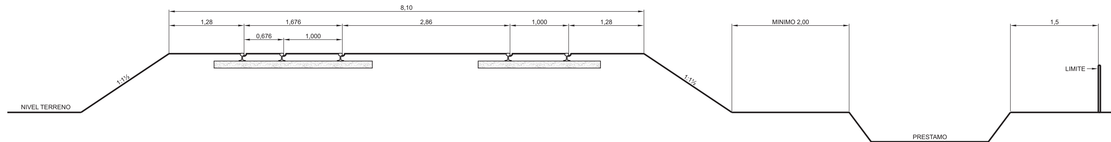
SECCION TRANSVERSAL DE TERAPLEN
