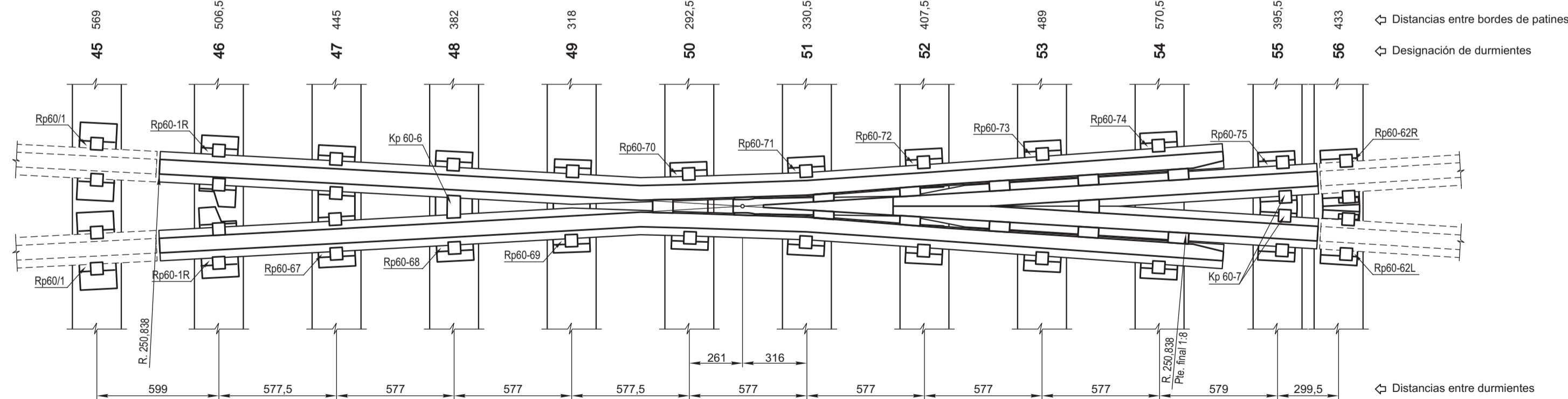
Colocación sobre durmientes de madera Esc. 1:20
