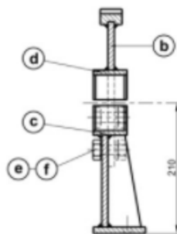
CORTE AA (S/Escala)
