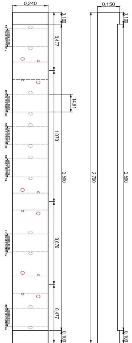
Detalle de durmiente para TROCHA MIXTA Escala: 1:10 Medidas en m
