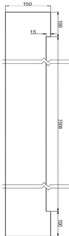
Detalle de fresa Escala: 1:5 Medidas en mm
