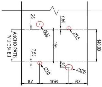
Detalle de perforaciones para fijaciones Escala: 1:5 Medidas en mm
