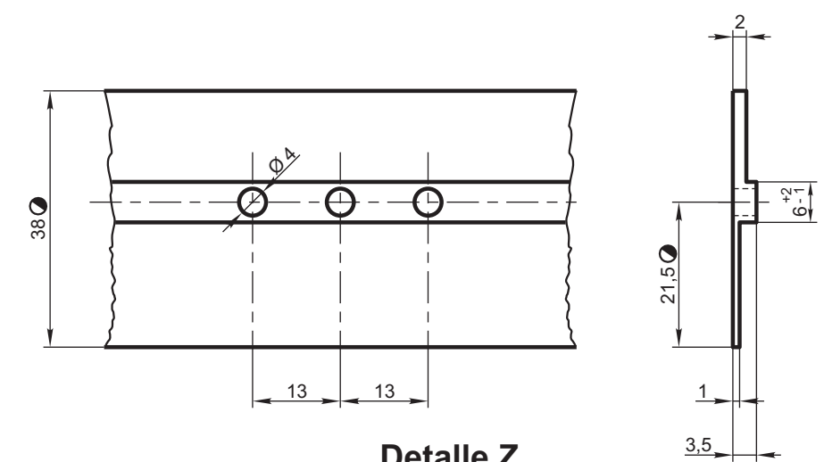
Detalle Z Esc. 1:1
