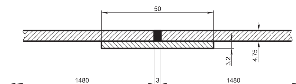
CORTE A-A Esc. 1:1
