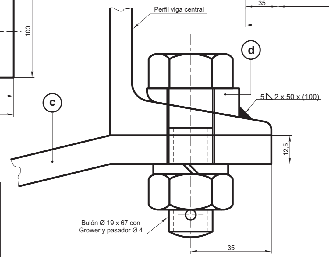
Detalle sujeción soporte yugo Esc. 1:1
