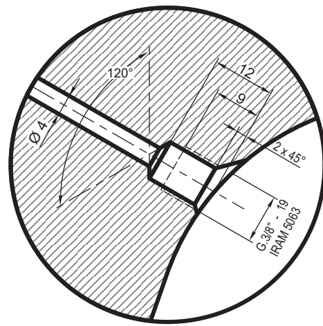
DETALLE "1" (Esc. 1:1)
