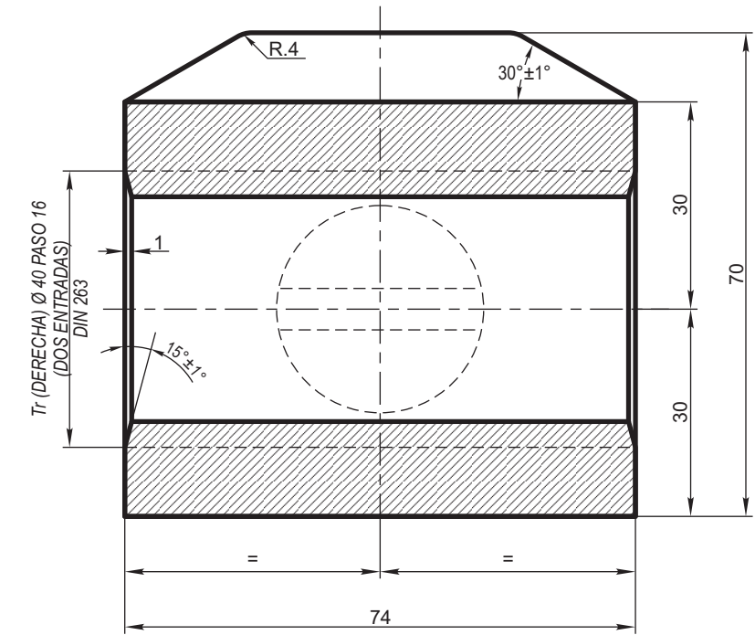
CORTE A-A
