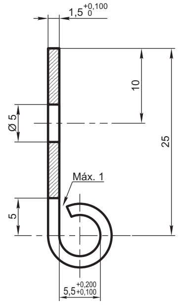
CORTE E-E (Esc. 2:1)
