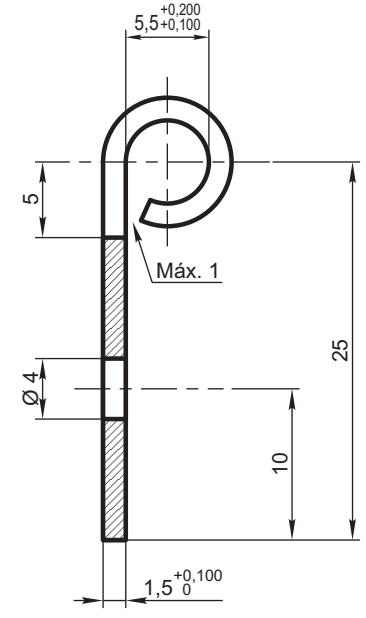
CORTE F-F (Esc. 2:1)
