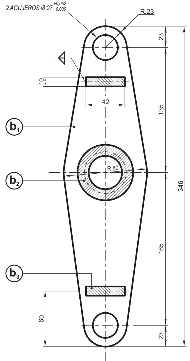
CORTE A-A
