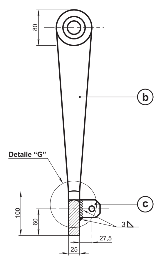
CORTE F-F
