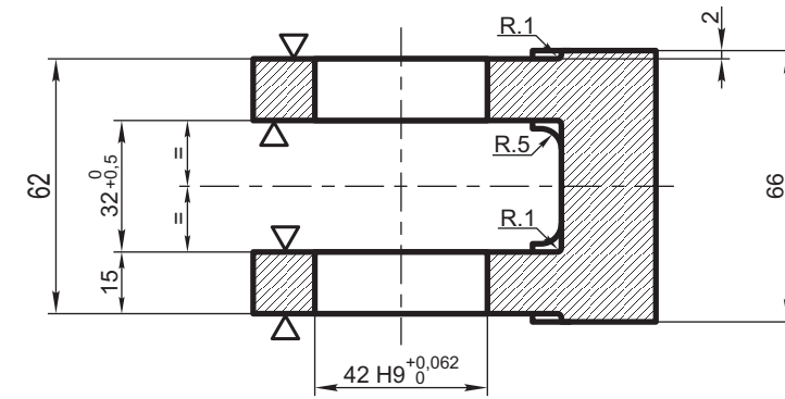
CORTE F-F
