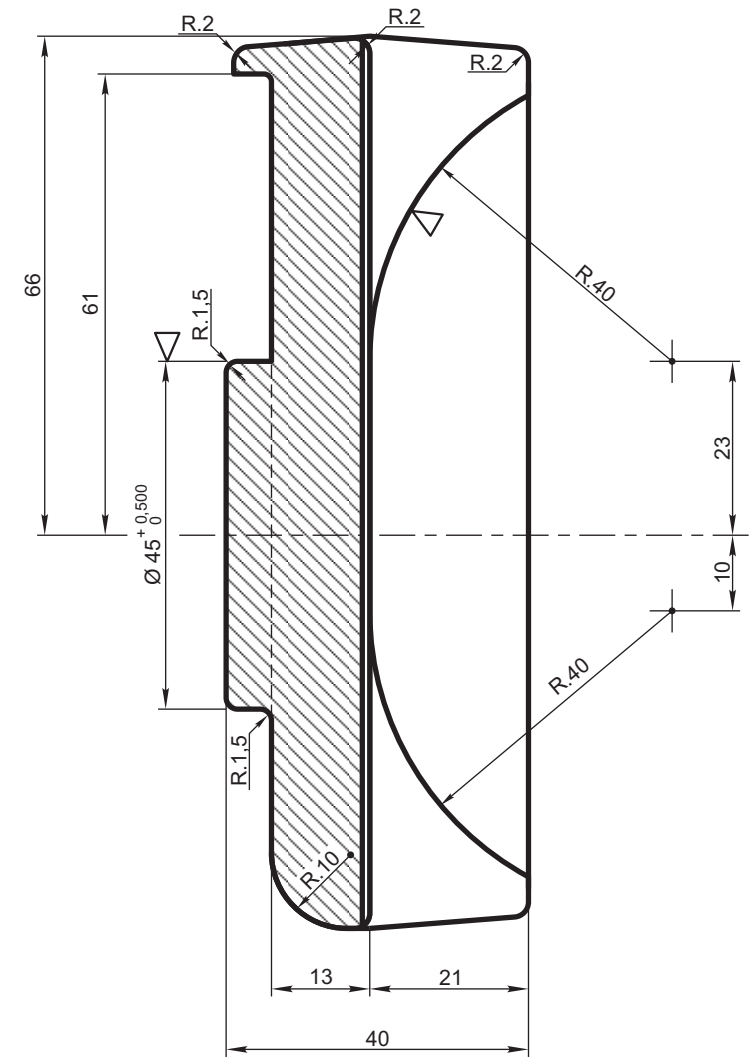
CORTE A-A
